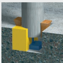
Prefabricirani stupovi
