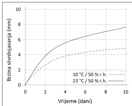
Dijagram 1: Brzina stvrdnjavanja Sikaflex®-529 Evolution
