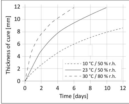
Dijagram 1: Brzina stvrdnjavanja SikaTack® Panel
